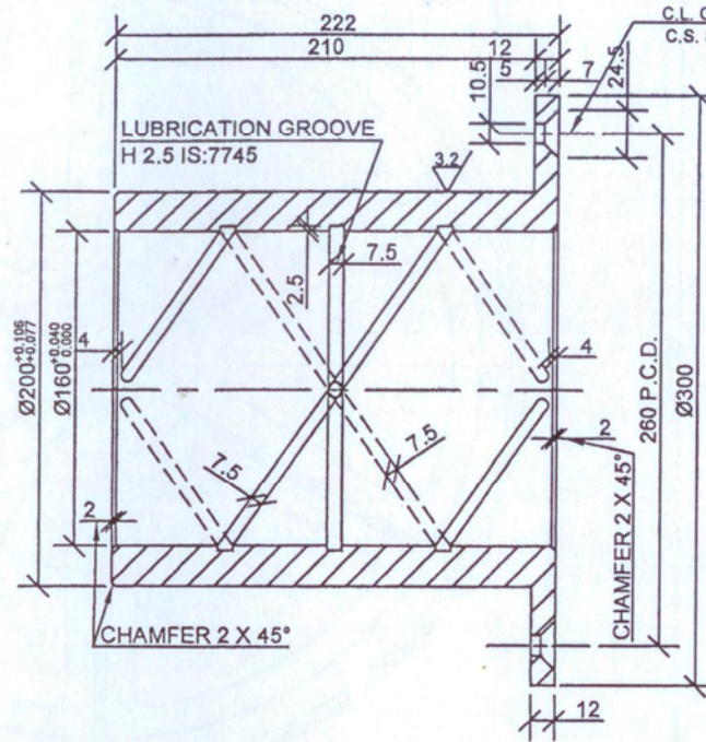
SECTION - DD
