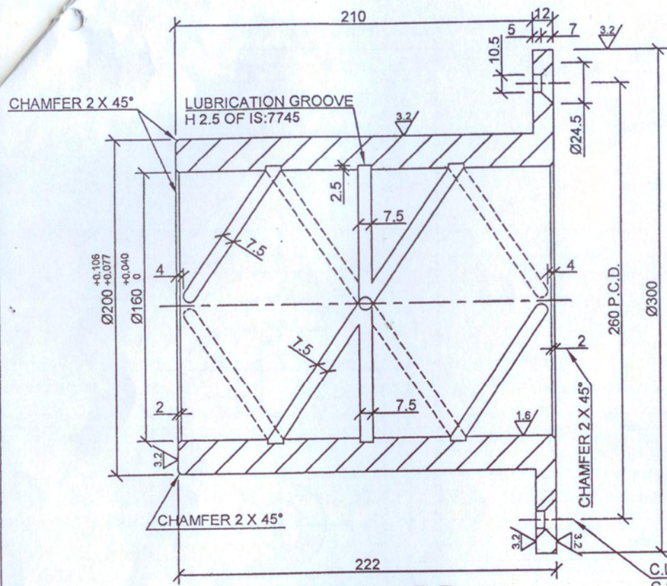
SECTION - DD
